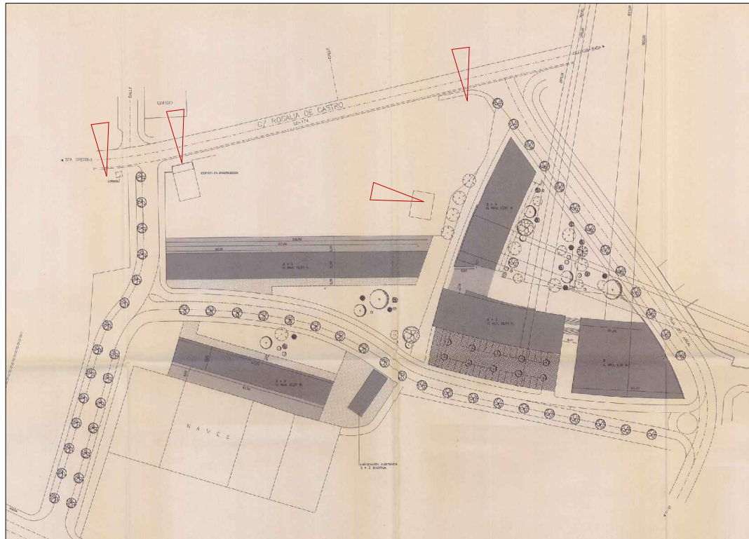
PLAN ESPECIAL DE REFORMA INTERIOR DE LA UE-17 PLANO N° 3. ALINEACIÓN
