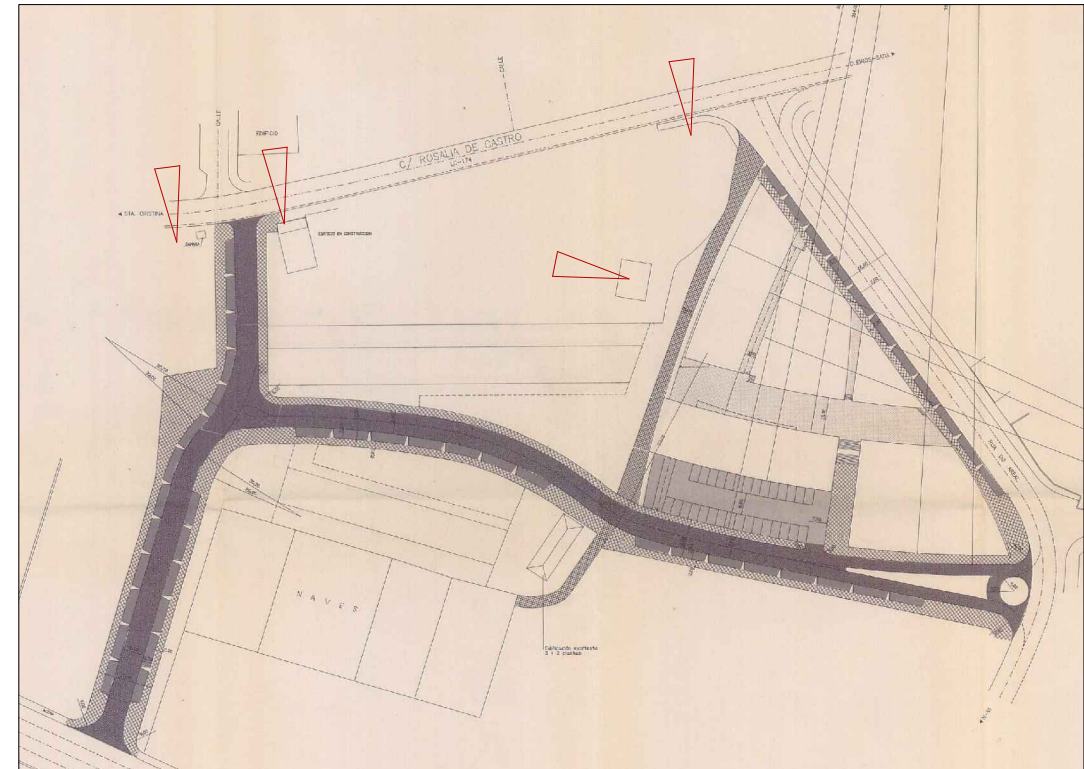
PLAN ESPECIAL DE REFORMA INTERIOR DE LA UE-17 PLANO N° 6. SISTEMA VIARIO
